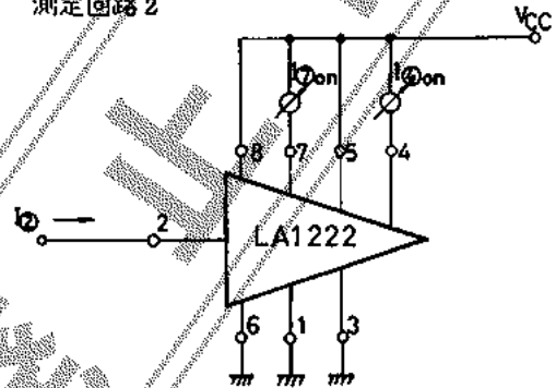
測定回路 2
