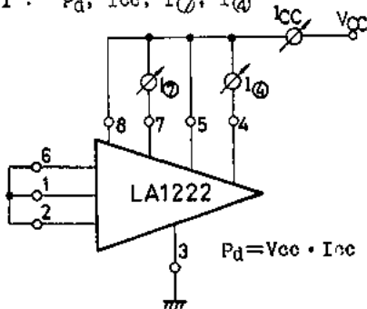
測定回路 1 : P_d , I_{cc} , I_{QI} , I_{QII}
